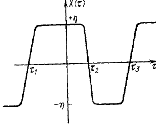
Рис. 3: Многоинстантонная конфигурация
